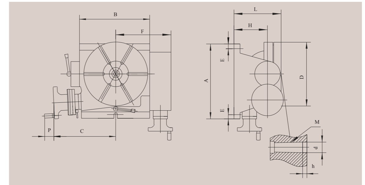
1004-0100...0400, 1004 (TSK) 系列回转工作台安装尺寸参数: Installation sketch and dimensions
